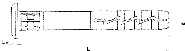
Manșon FX-..K..
