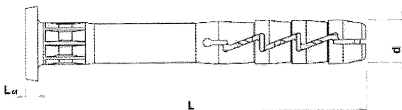
Manșon FX-..C..
