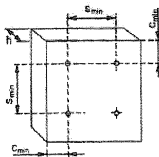
Diagramă spațiere
