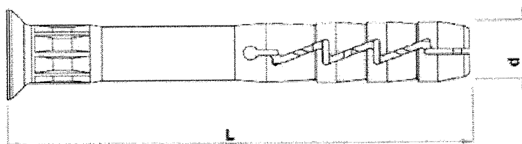
Manșon FX-..L..
